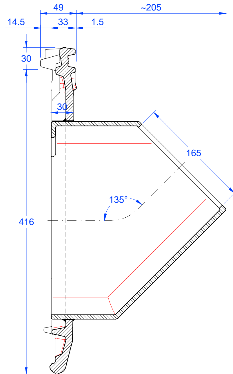
Schnitt B-B
