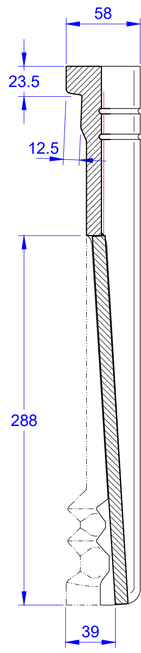
Schnitt A-A
