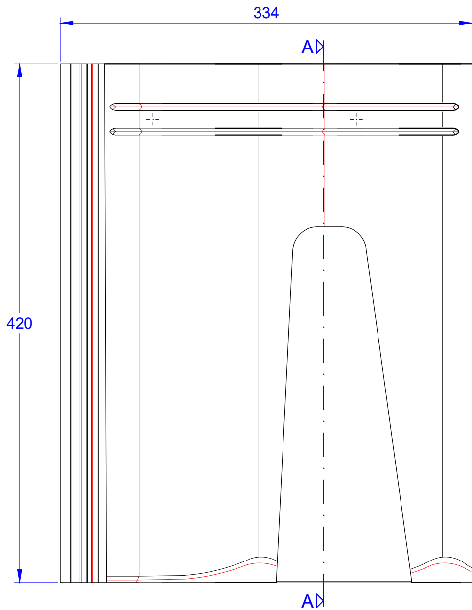
Ansicht
