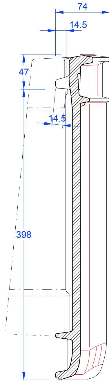
Schnitt B-B
