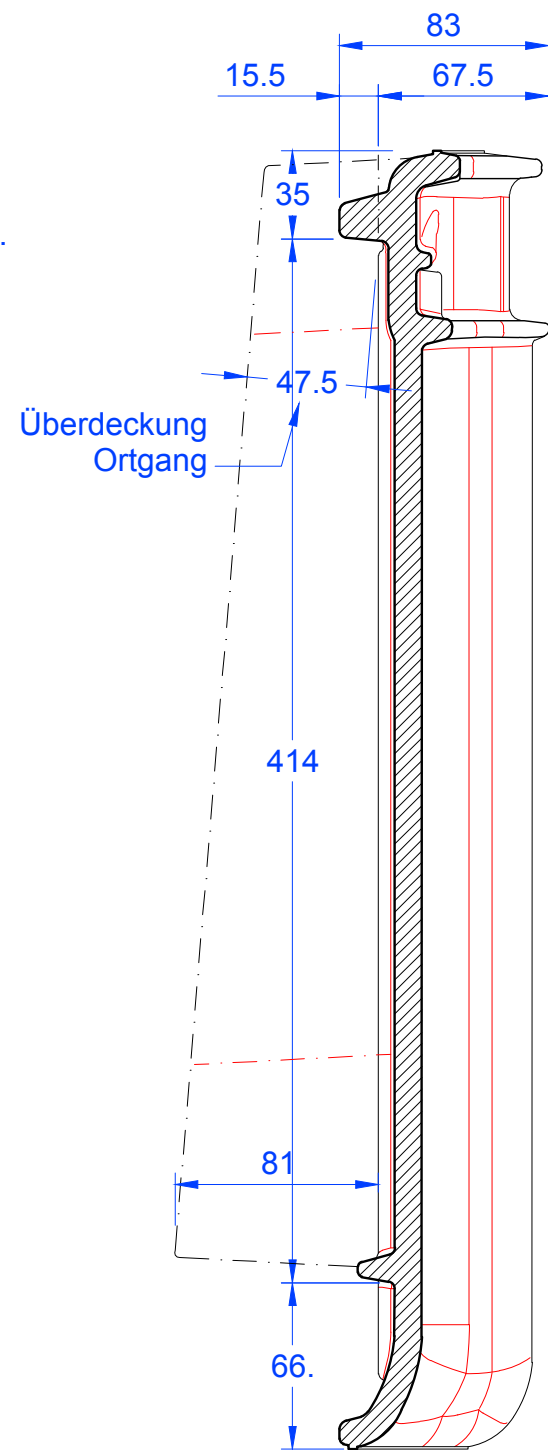
Schnitt B-B
