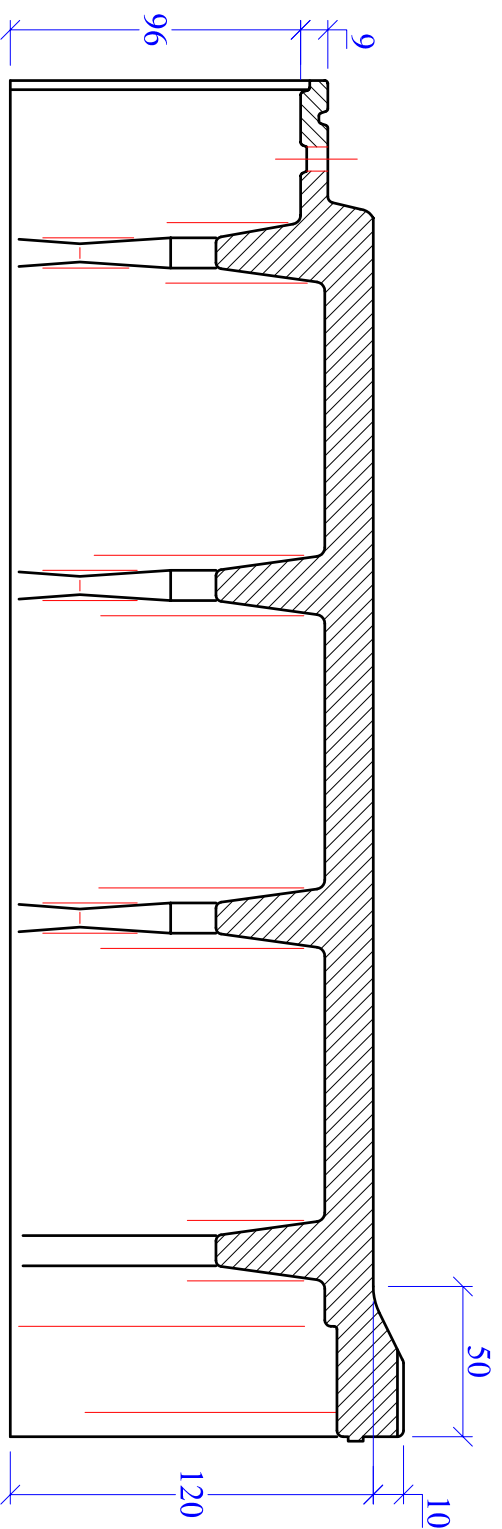
Längsschnitt
